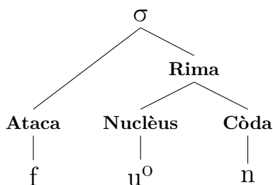
FIGURA 4.2 – Representacion desvelopaa (arbre) de l'estructura sillabica
