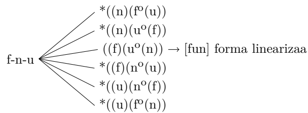
FIGURA 4.3 – Ilustracion dau processús de d’estructuracion de la sillabacion : lo material fonologic inèrte f-n-u es organizat per formar una forma linearizaa (doncas viabla) (f)(u°(n)).
